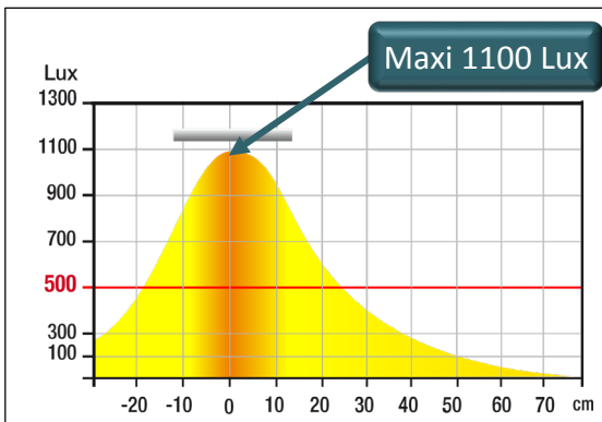
Mesure en Lux sur le plan de travail en vue de profil à 35 cm:
