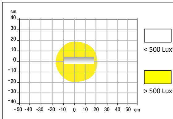
Mesure en Lux sur le plan de travail en vue de dessus à 35 cm:
